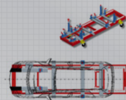
Exemple d'utilisation avec Sevenne en combinaison avec MZ ou MZ+. Measuring with Sevenne and MZ or MZ+
